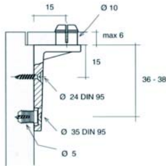
Rugwandklem type 57.0570
