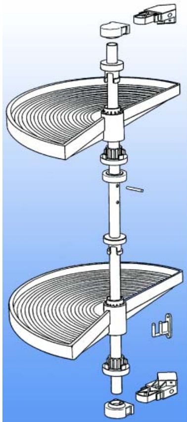
Type ST 522 voor montage op stijl
