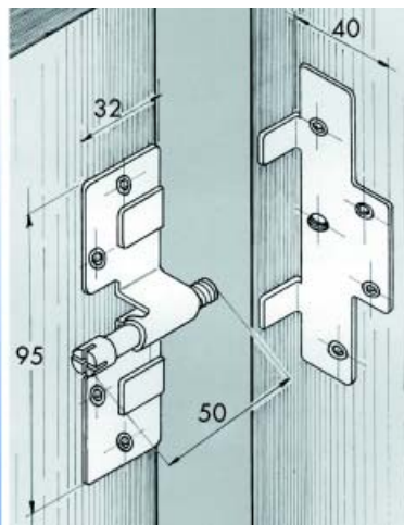
Hoekverbinding type 0561.01.098
