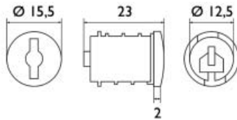
Gelijksluitende series - cilinder met 2 sleutels
