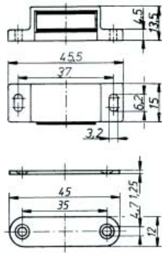
Magneten type 272/2L
