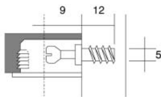
Stift voor Modulfix kastverbindingen - euroschroef
