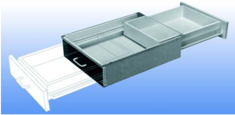
Geleider voor dubbelzijdig uittrekbare laden type BAX 20
