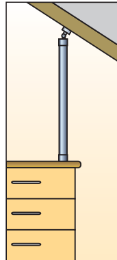
Asbuis en adapter voor schuine plafonds, van het werkblad tot aan de dakschuimte.
